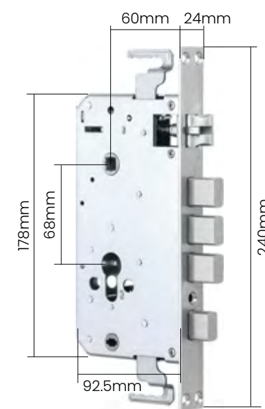
6068 (24×240mm) Top & Bottom Hooks
